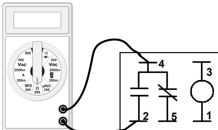
TESTING FAN RELAY
